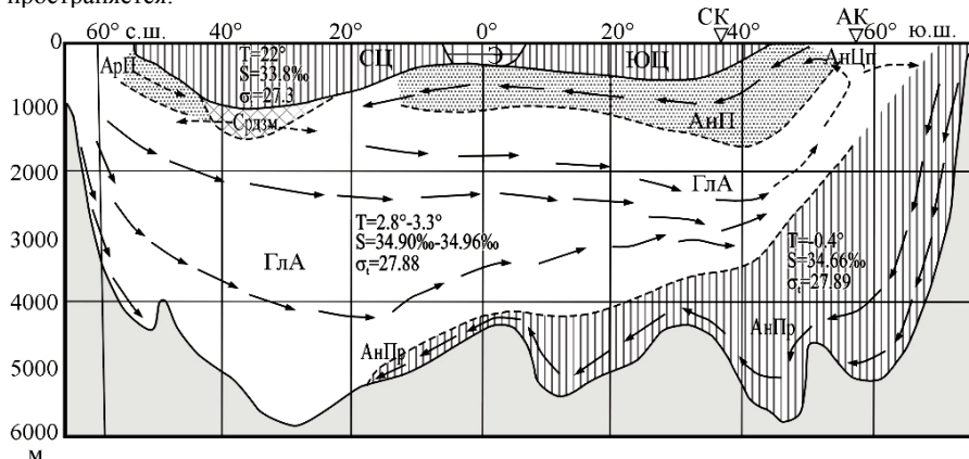
Рис. 36. Схема водных масс на меридиональном разрезе через Атлантический океан. АнПр - антарктическая придонная; ГЛА - североатлантическая глубинная и придонная; АнЦп - антарктическая циркумполярная; Срдзм - средиземноморская; СЦ - северная центральная; ЮЦ - южная центральная; АнП - антарктическая промежуточная; АрП - североатлантическая промежуточная; Э - экваториальная; АК - антарктическая конвергенция; СК - субтропическая конвергенция.
