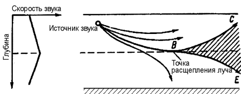
Рис. 17. Рефракция звуковых лучей при увеличении скорости звука в поверхностном слое и ее убывании ко дну (изменение положительной рефракции в верхнем слое на отрицательную в нижележащих слоях).
