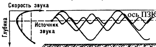
Рис. 18. Подводный звуковой канал
