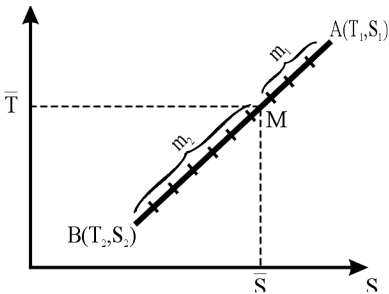
Рис. 29. T,S-соотношение и прямая смешения двух водных масс
