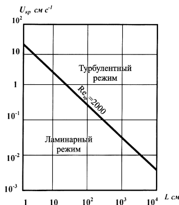
Рис. 6. Зависимость критической скорости ламинарного течения от его характерного линейного масштаба при Re_{кр}=2000
