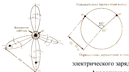
Рис.3. Молекула воды: ● - ядро атома кислорода О или водорода Н, х - электрон, общий для атомов кислорода и водорода, (+) и (-) области результирующего
