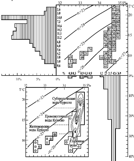
Рис. 35. Статистическая Т,S-диаграмма объемов водных масс Восточно-Китайского моря
