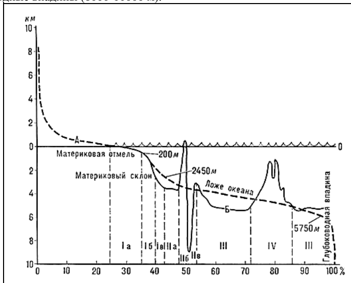
Рис. 2. Гипсографическая кривая (А) и обобщенный профиль дна океана (Б). (I - подводная окраина материков, II - переходная зона, III - ложе океана, IV - срединно-океанические хребты).
