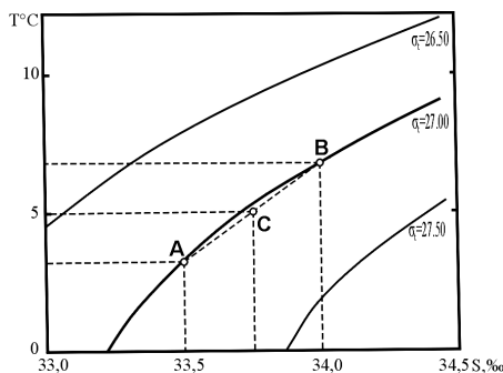
Рис. 5. Уплотнение при смешении двух объемов морской воды
