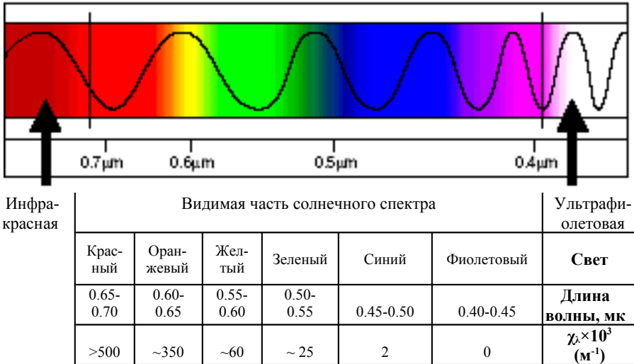
Показатели поглощения \chi_\lambda волн видимой части солнечного спектра
