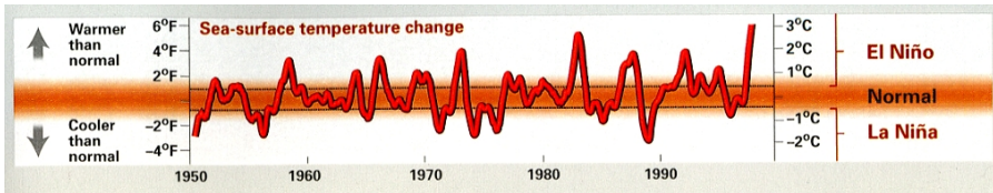
Рис. 23. Изменения поверхностной температуры воды в центральной экваториальной части Тихого океана с 1950 по 1998 гг. (National Geographic, march 1999)
